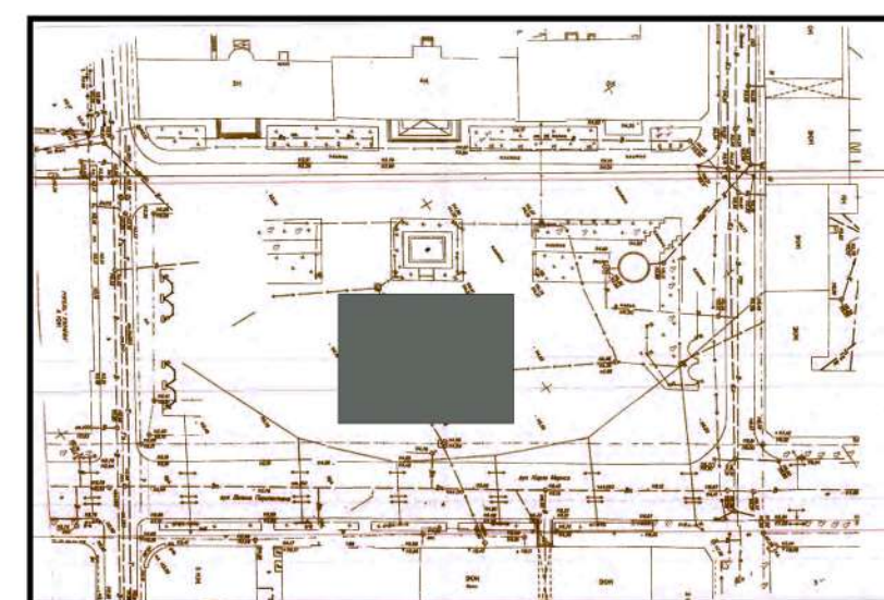
ГЕНПЛАН
